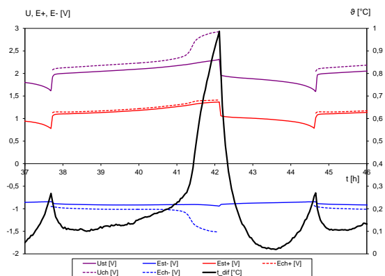
Obr. 6: Závislost teploty, napětí a potenciálů u vybíjení a pulzního nabíjení 1. článku (druhý experiment)
