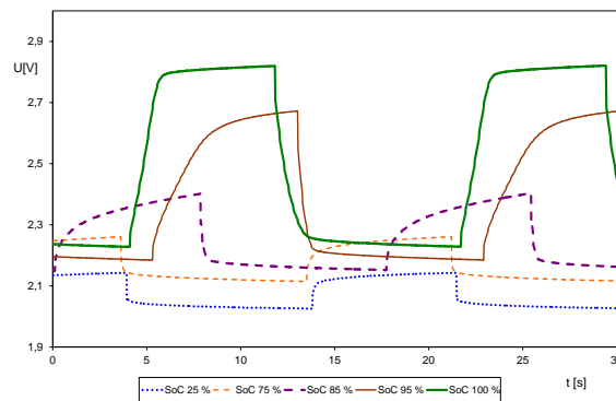
Obr. 4: Napěťové průběhy pro různé stupně nabití při pulzním nabíjení 2. článku. (první experiment)
