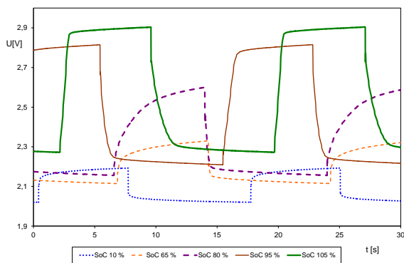
Obr. 2: Napěťové průběhy pro různé stupně nabití při pulzním nabíjení 1. článku. (první experiment)
