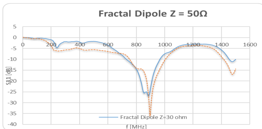
Obrázek V. Závislost parametru S_{11} fraktál-dipólové antény na frekvenci
