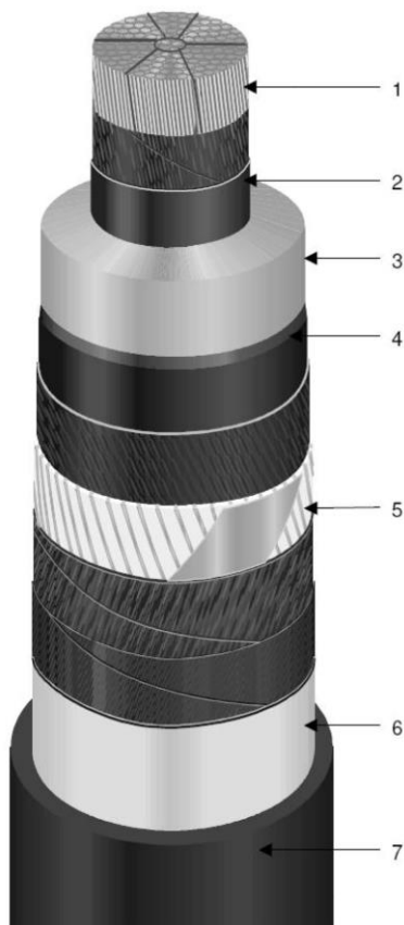
Obr. 1: Fázový kabel
