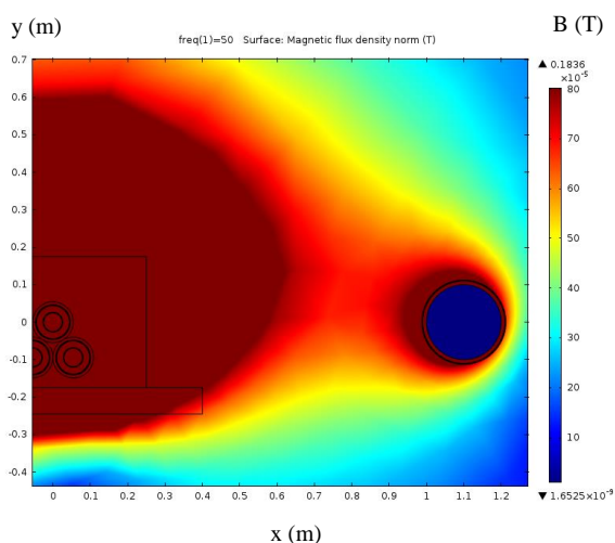
Obr. 5: Rozložení magnetického pole pro vzájemnou vzdálenost 1,1 m - Ocel 2 ( \mu_r=200 )
