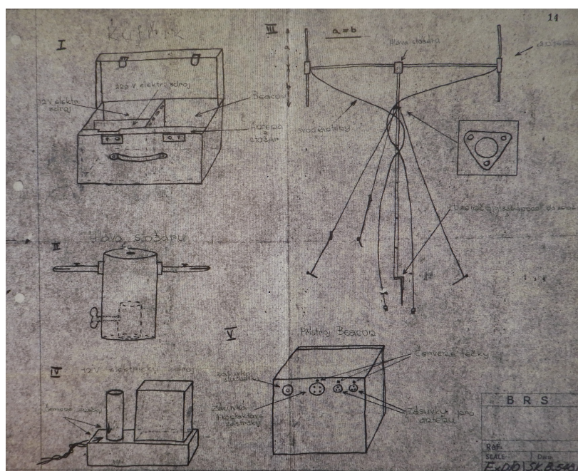
Příloha č. 8: Návrh naváděcího zařízení Rebeca Beacon z přípravy operace Out Distance. 414
