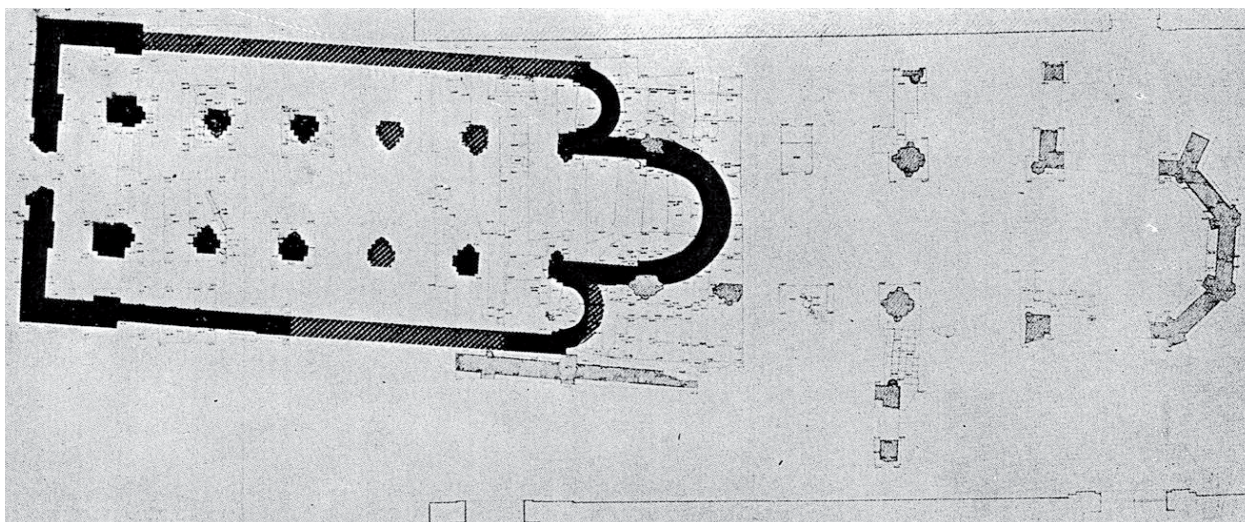
Obr. 1. Litomyšl. Půdorysná dispozice románské baziliky Panny Marie a gotické přestavby. Podle Reichertová – Merhautová-Livorová 1966, 319. – Abb. 1. Litomyšl. Grundriss und Disposition der romanischen Basilika der Jungfrau Maria und gotischer Umbauarbeiten. Nach Reichertová – Merhautová-Livorová 1966, 319.
