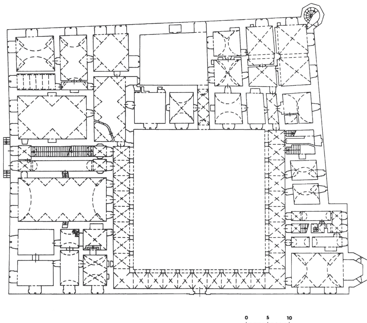
Obr. 2. Litomyšl. Přízemí renesančního zámku. Podle Muk – Šrámková, 1985, 286. – Abb. 2. Litomyšl. Erdgeschoss des Renaissance-Schlusses. Nach Muk – Šrámková, 1985, 286.
