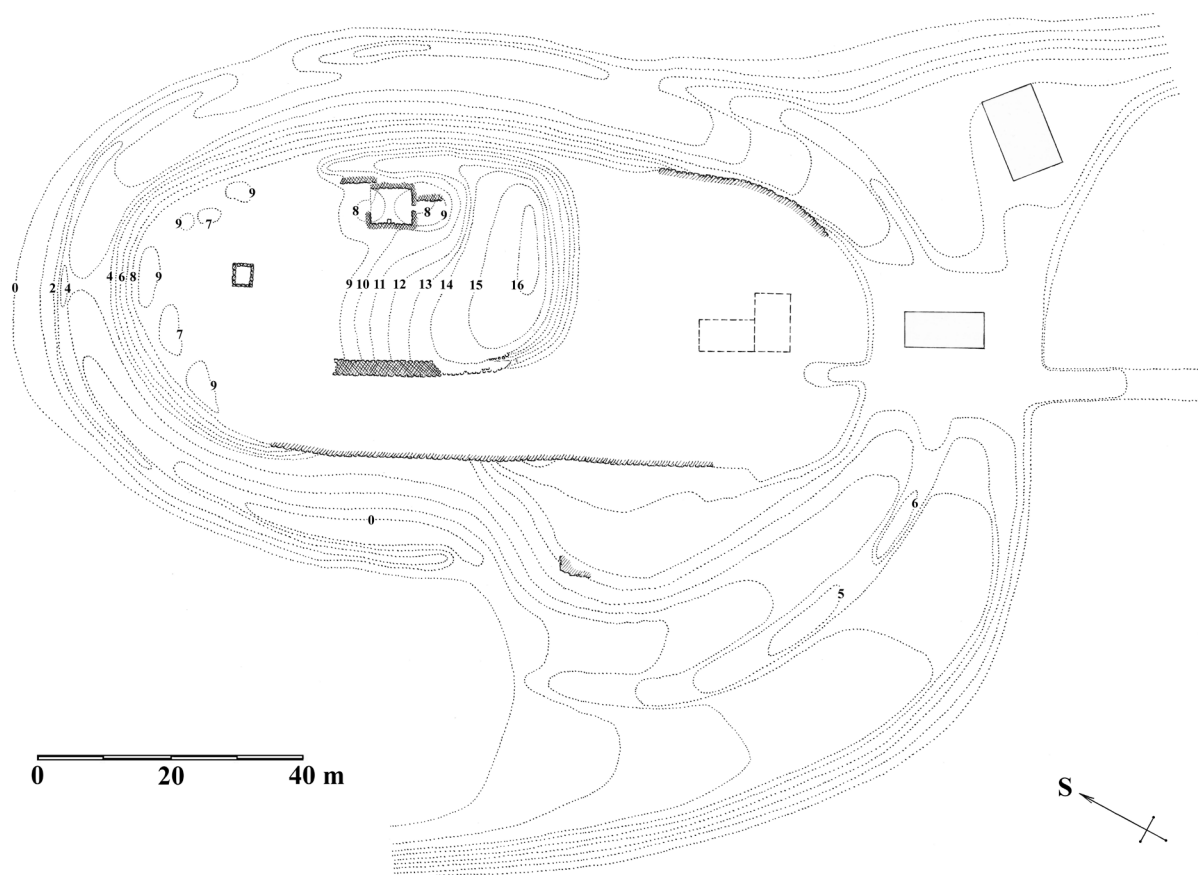
Obr. 4. Skica relikvů hradu Ronov (Trzcinec, woj. Jeleniogórskie, Polsko) z roku 1987. Zaměření F. Gabriel – J. Panáček, měřeno pásmem. – Abb. 4. Die Skizze der terrainrelikten der Burg Rohnau (Trzcinec, woj. Jeleniogórskie, Polen) aus dem Jahre 1987. Vermessung F. Gabriel – J. Panáček (Bandmessung).
